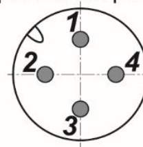
Цоколевка разъема
