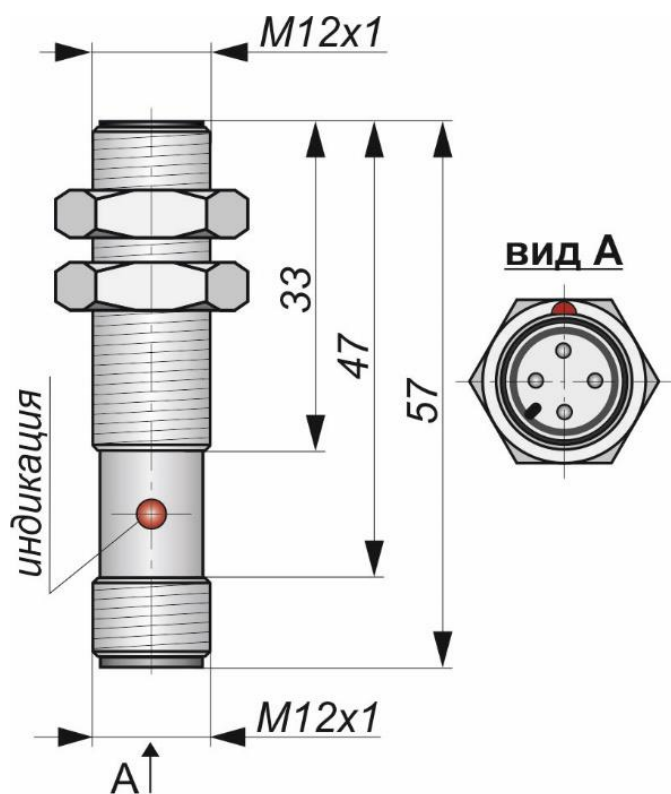
Габаритный чертеж
